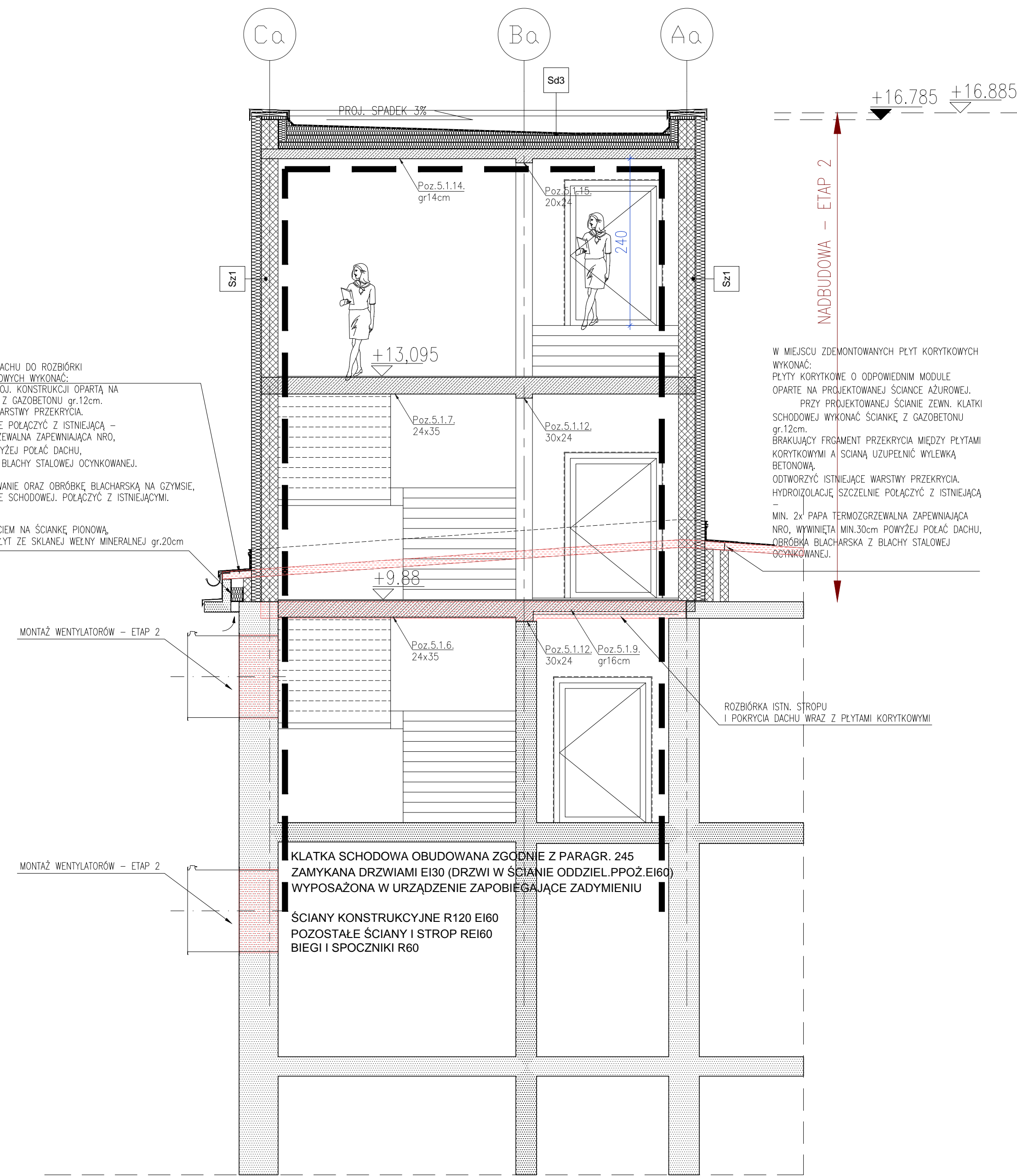
PRZEKRÓJ C'-C'
