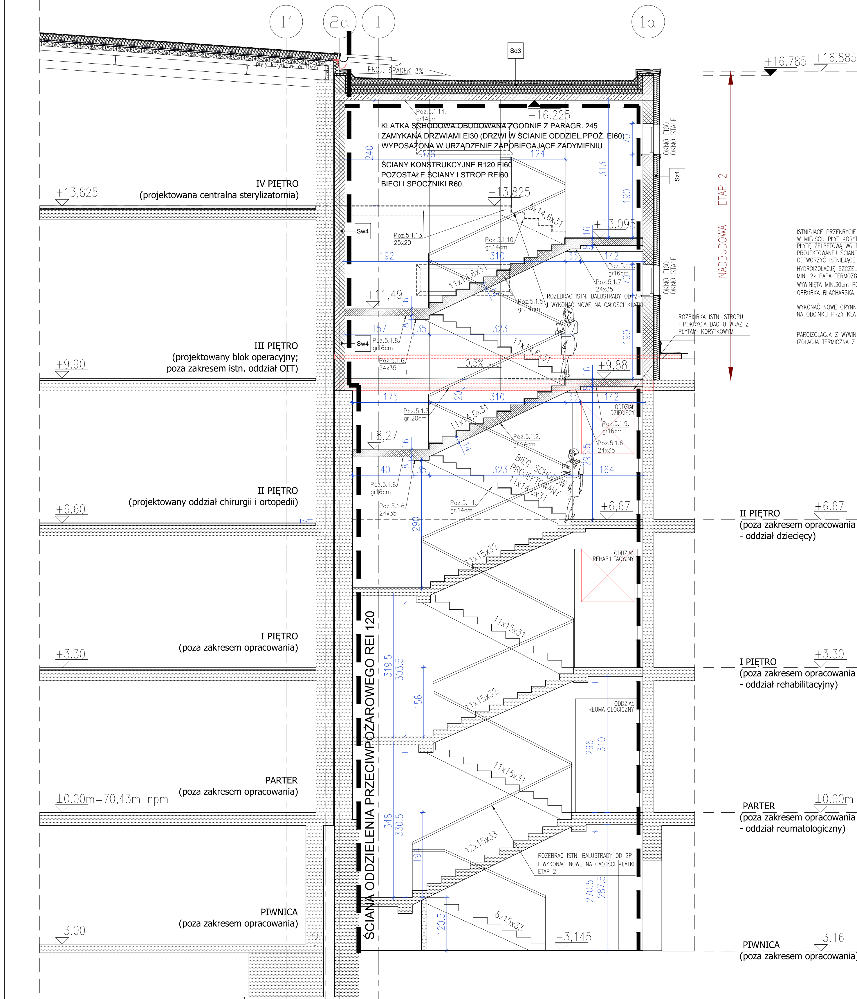
PRZEKRÓJ C'-C'
