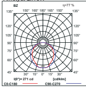
Ametyst 2x18W
