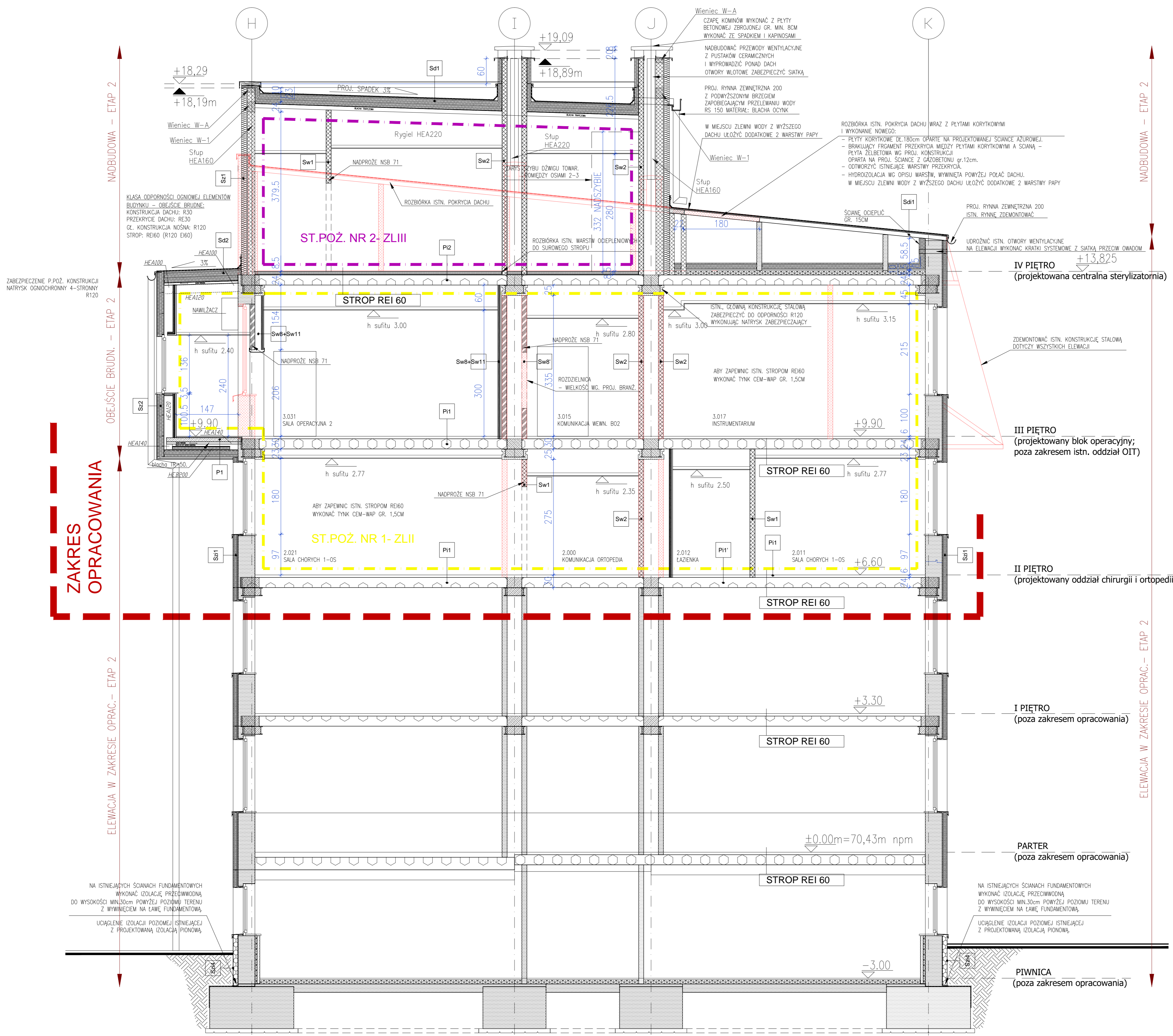
PRZEKRÓJ A-A
